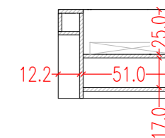
Przekrój A-A
