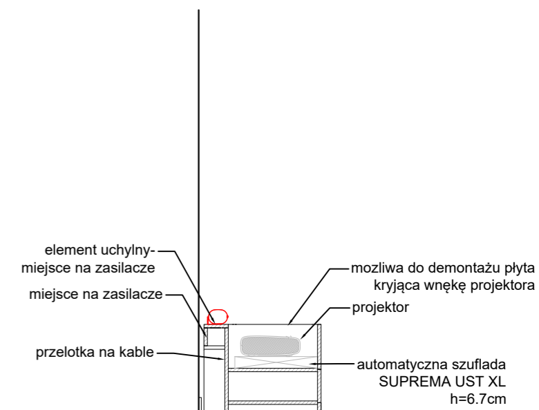
Przekrój A-A
