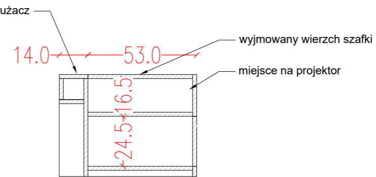
Przekrój A-A
